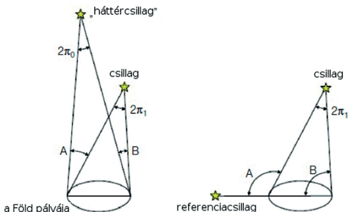
1. ábra. A parallaxis mérésének elve. Balra a relatív parallaxis, jobbra az abszolút parallaxis meghatározásának szemiatikus ábrázolása látható (URL1)
